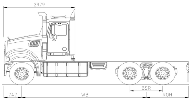
6x4 Day Cab Rigid
